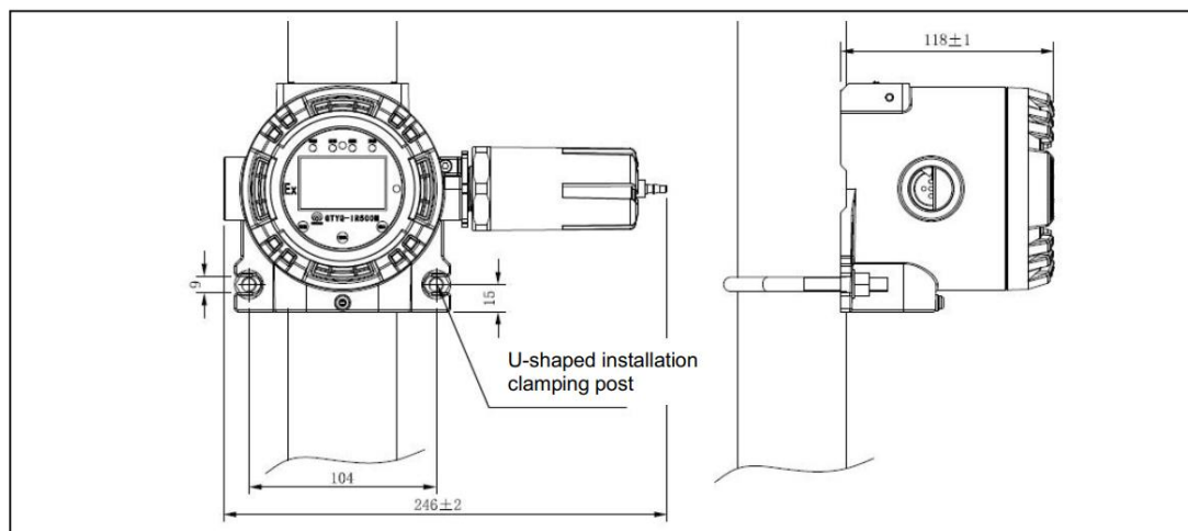
Рисунок 10 - Установка на вертикальной трубе
