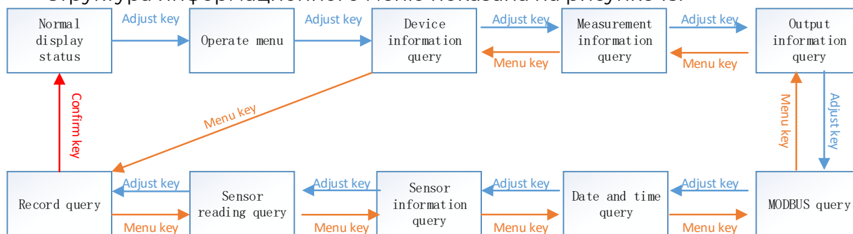
Рисунок 15 - Информационное меню газоанализатора
