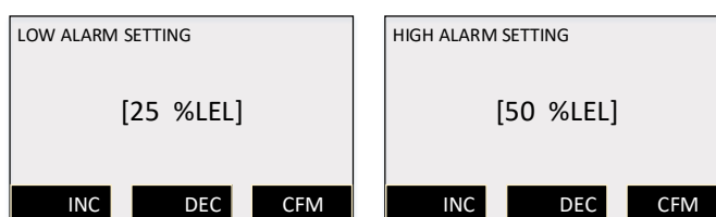
Рисунок 22 - Меню установки порогов тревог
