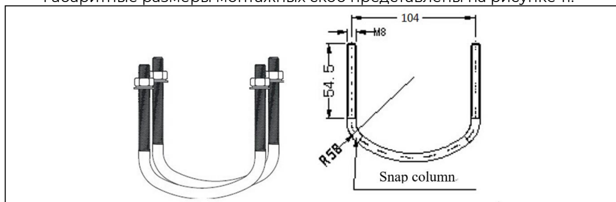
Рисунок 11 - Габаритные размеры монтажных скоб
