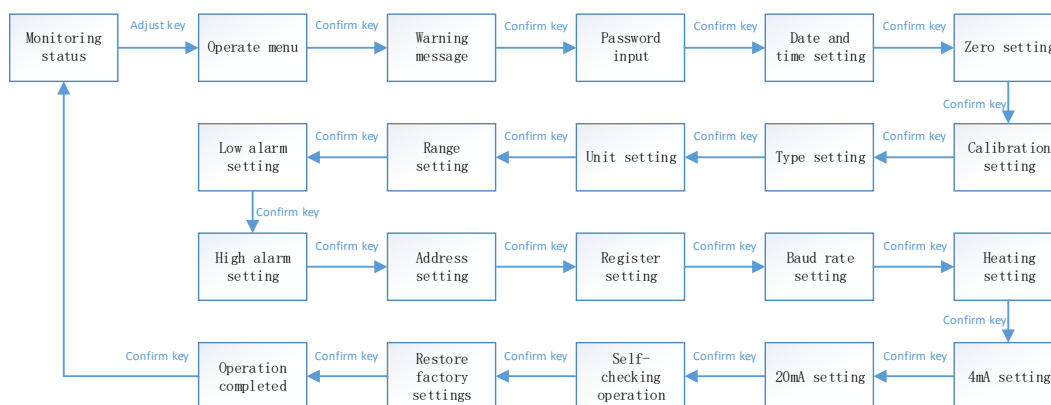
Рисунок 16 - Меню параметров газоанализатора
