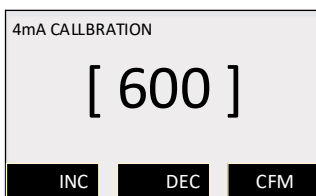
Рисунок 26 - Меню калибровки токового выхода 4 мА
