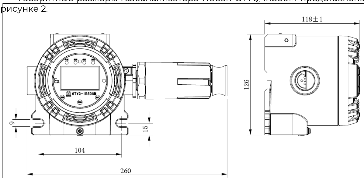
Рисунок 2 - Габаритные размеры газоанализатора Nuoan GTYQ-IR500M, мм
