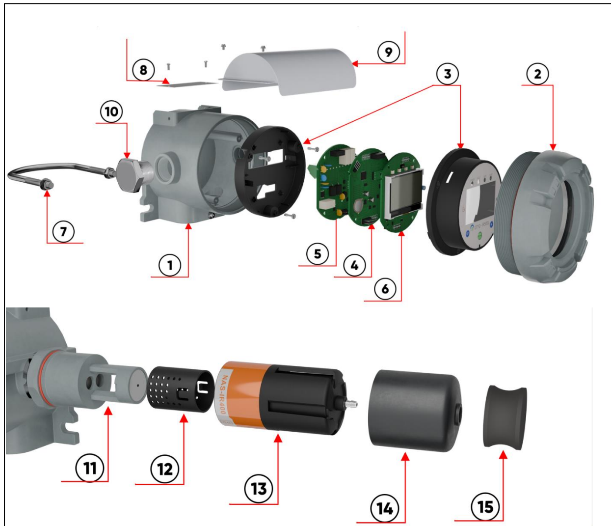
Рисунок 3 - Конструкция газоанализатора Nuoan GTYQ-IR500M
