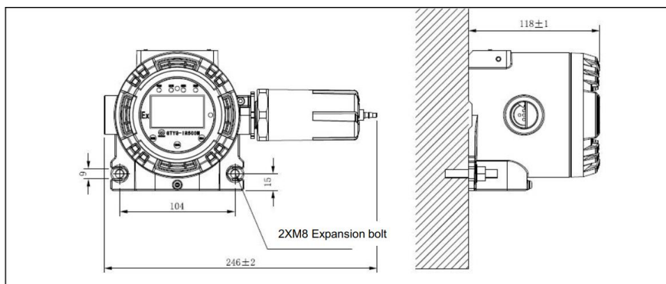
Рисунок 12 - Монтаж на стене
